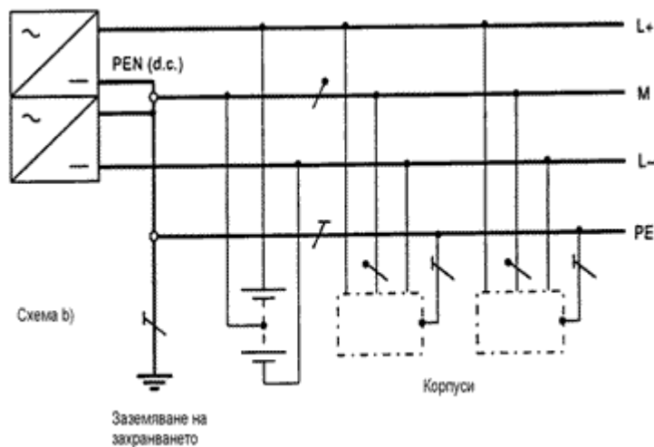
Фиг. 6. Схема TN-S при постояннотокови мрежи
