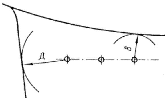
Фиг. 13. Минимални разстояния между тоководещи части на различни вериги, разположени в различни равнини, при обслужване на по-нискостоящата верига и наличие на напрежение на по-високостоящата верига.
