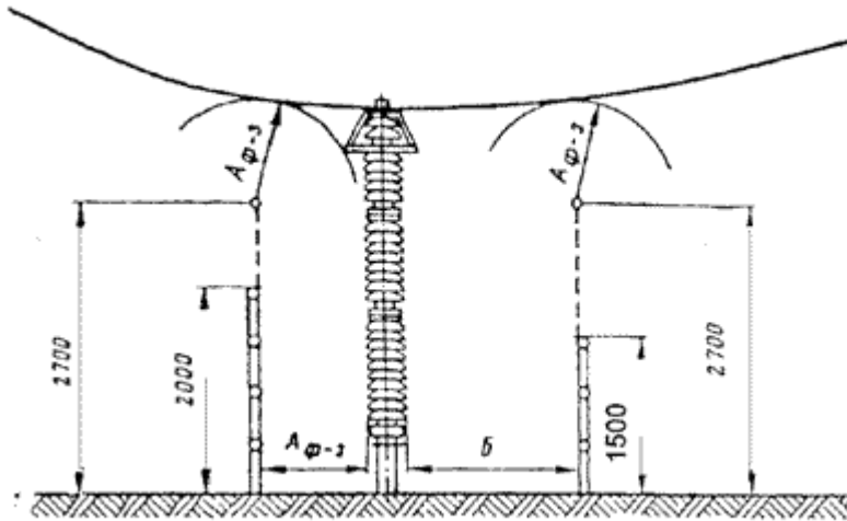
Фиг. 10. Минимални разстояния от тоководещи части и от елементи на изолятори, които се намират под напрежение, до постоянни вътрешни огради.
