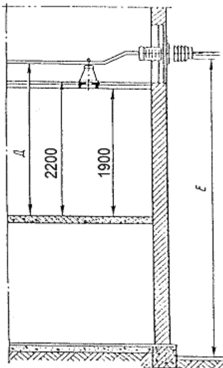
Фиг. 21. Минимални разстояния от неограничени тоководещи части и от долния ръб на изолаторите до пода; светла височина на коридора в ЗРУ; минимални разстояния от неограничени линейни изводи от ЗРУ до терена във от територията на ЗРУ при липса на достъп на превозни средства под изводите
