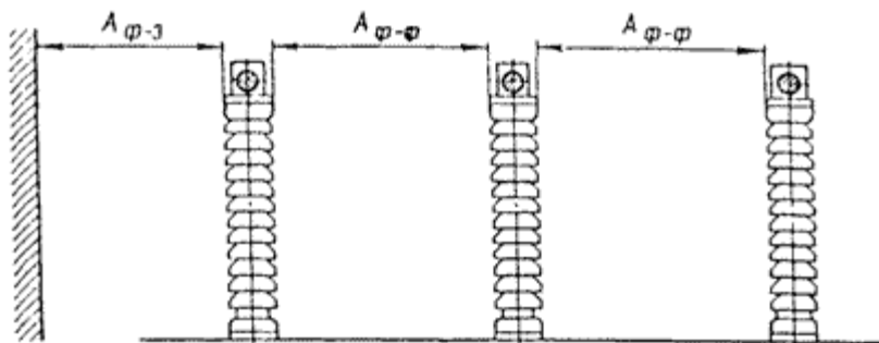
Фиг. 8. Минимални светли разстояния при твърди шини между тоководещи части и заземени части ( A_{\phi-3} ) и между тоководещи части на различни фази ( A_{\phi-\phi} ).
