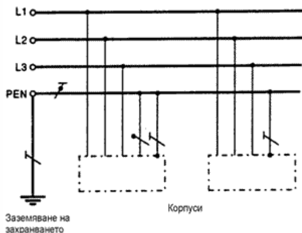
Фиг. 3. Схема TN-C
