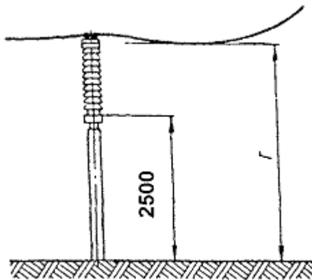
Фиг. 11. Минимални разстояния от неоградени тоководещи части и от долния ръб на изоляторите до земята.
