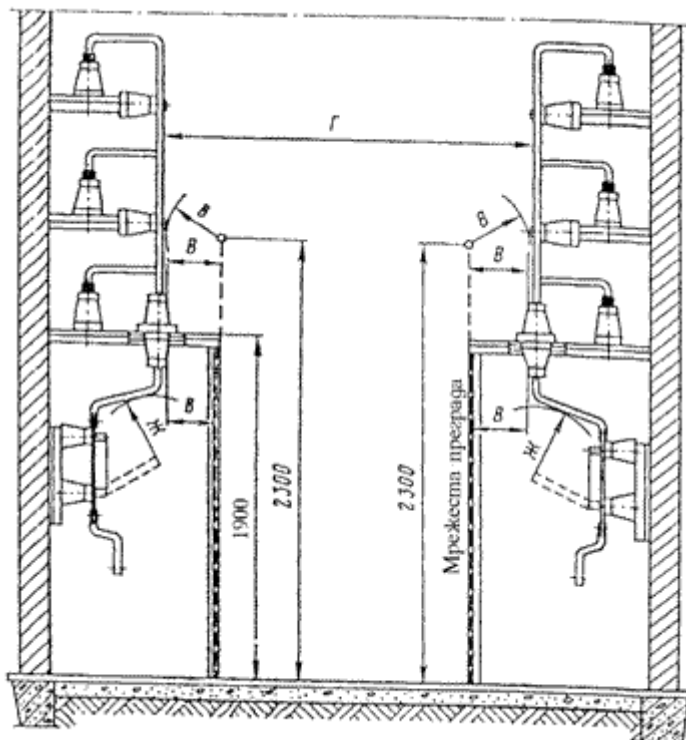
Фиг. 20. Минимални разстояния от тоководещи части до огради с мрежи и между неограничени тоководещи части на различни вериги
